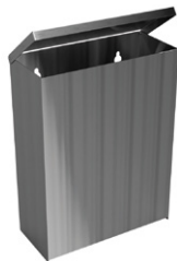
BM101915055 Koš odpadkový hranatý, závěsný Barva nerez mat Objem koše 6 l Rozměry (v × š × h) 300 × 205 × 100 mm
